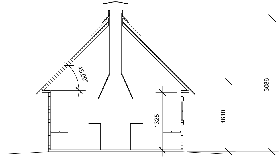
SEKTION (1:50)
