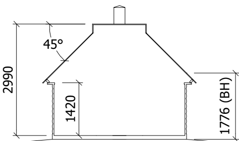
SEKTION A-A ( 1 : 100 )
