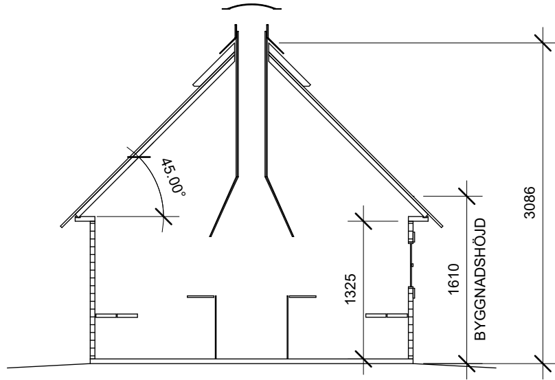
SEKTION GRILLKÅTA (1:50)
