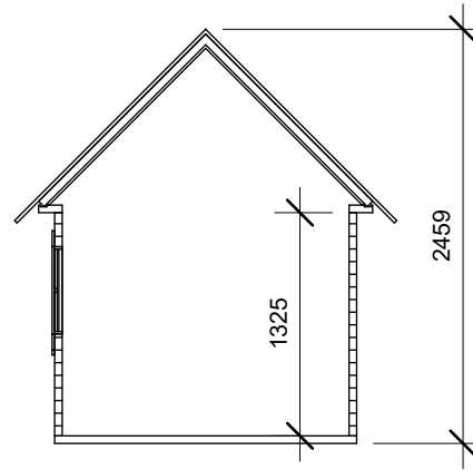
SEKTION BASTURUM (1:50)
