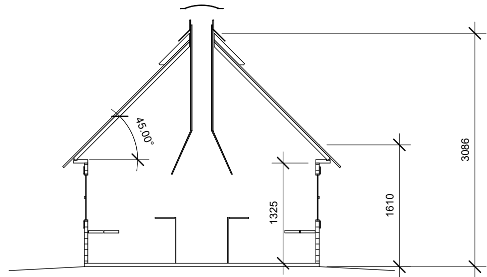
SEKTION (1:50)
